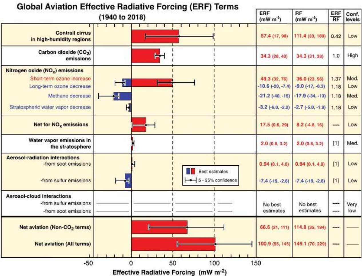
Einfluss klimawirksamer Emissionen. In rot wärmende und in blau kühlende Effekte unter Angabe von Konfidenzintervallen. 1
